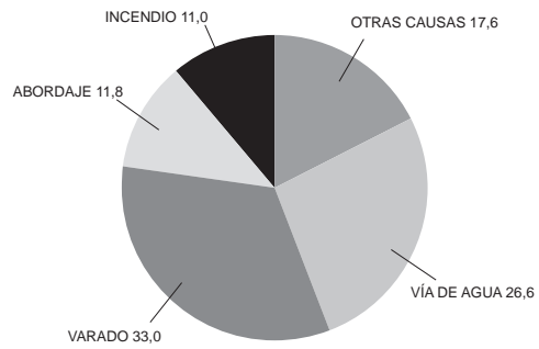
Buques afectados por accidente
