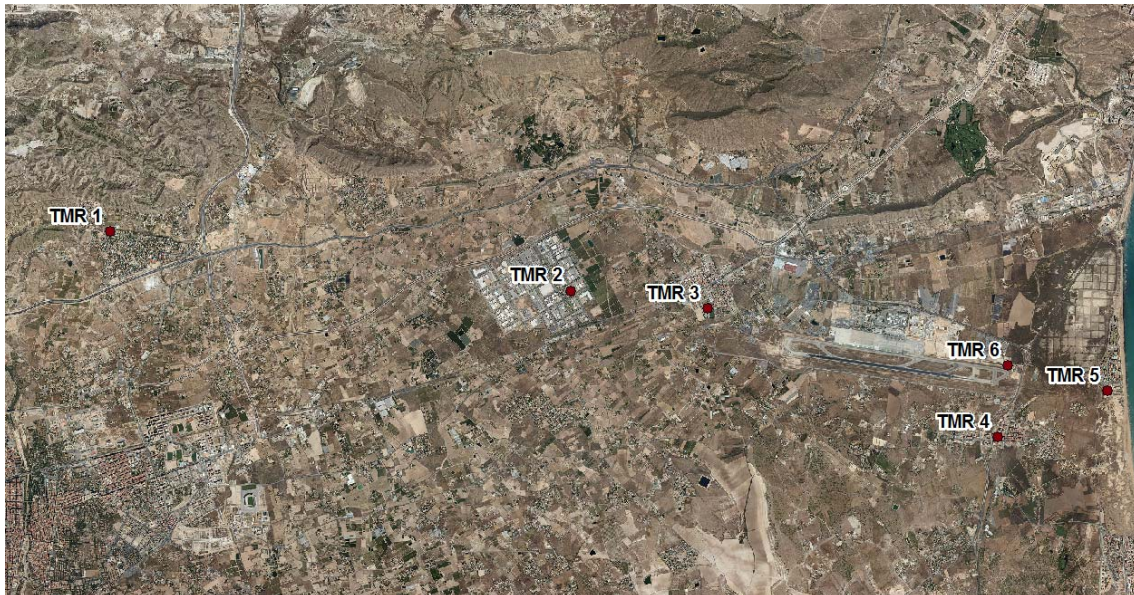
Ilustración 3. Localización de los TMR del Sistema de Monitorado de Ruido. Aeropuerto de Alicante-Elche
